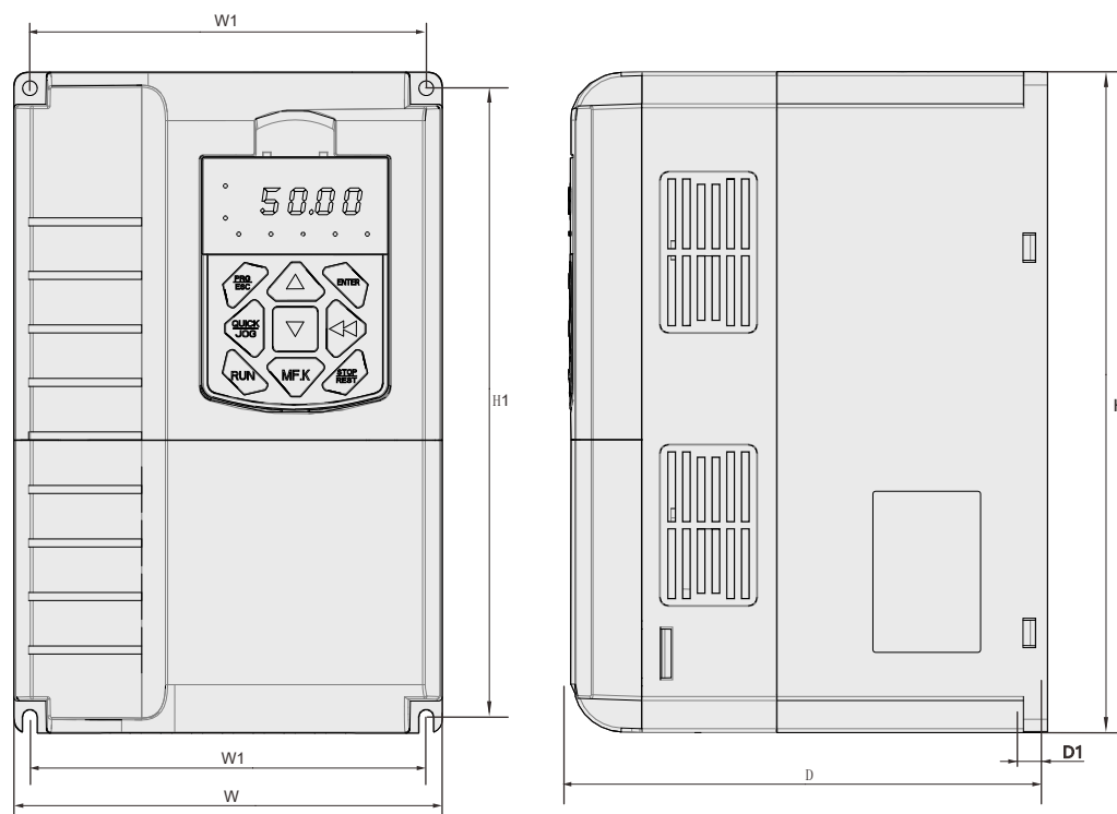
塑胶架构外形尺寸及安装尺寸示意图
