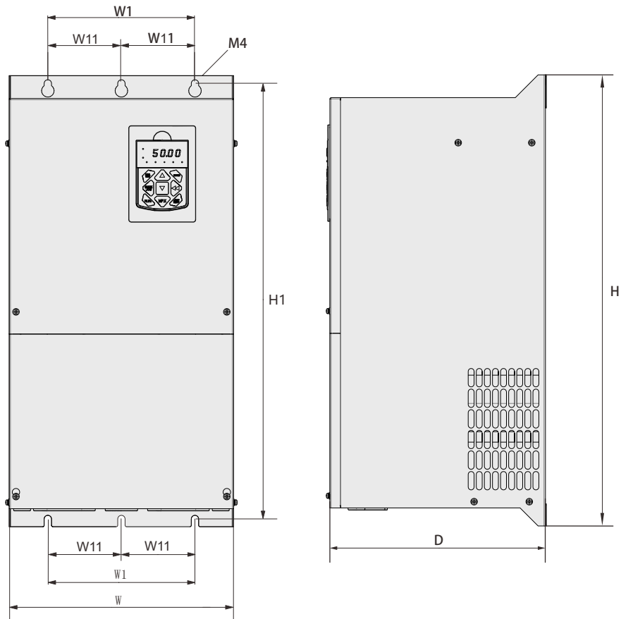
钣金架构外形尺寸及安装尺寸示意图
